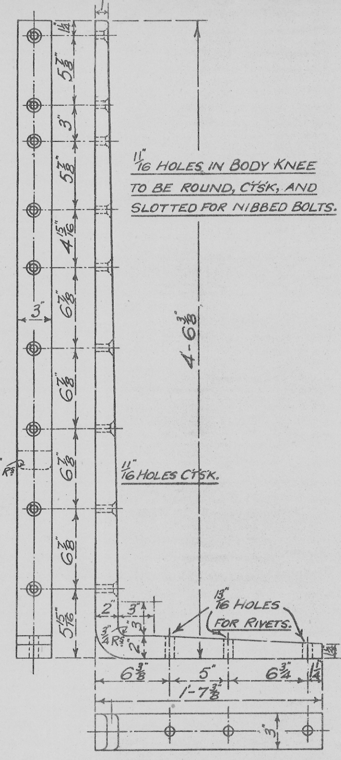
CORNER PLATE 2 PER SET
