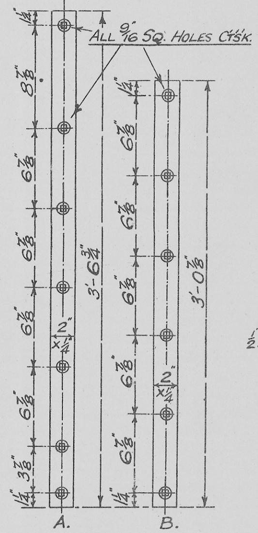
CORNER PLATE 2 PER SET
