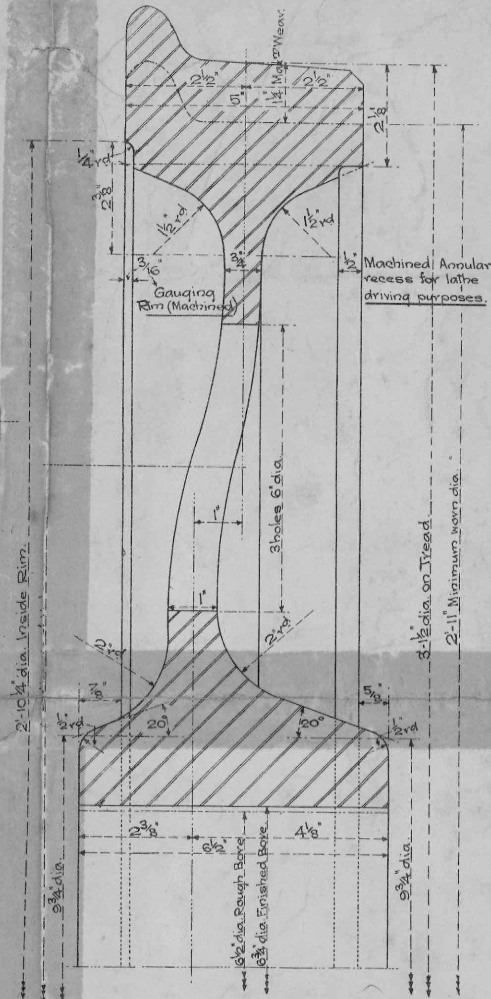
20 TON ORDY & TANK WAGONS.
